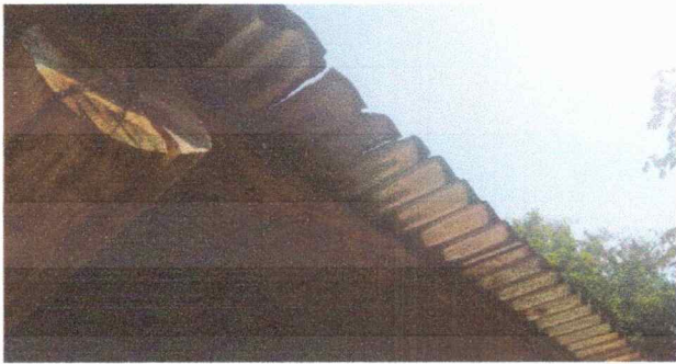
Foto 3: Se observa el deterioro del techo, la cual produce goteras en tiempos de invierno.
